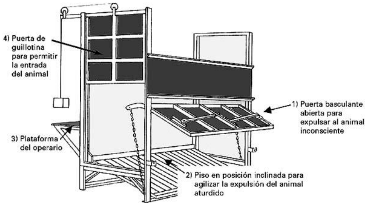
Diseño cajón de aturdimiento
