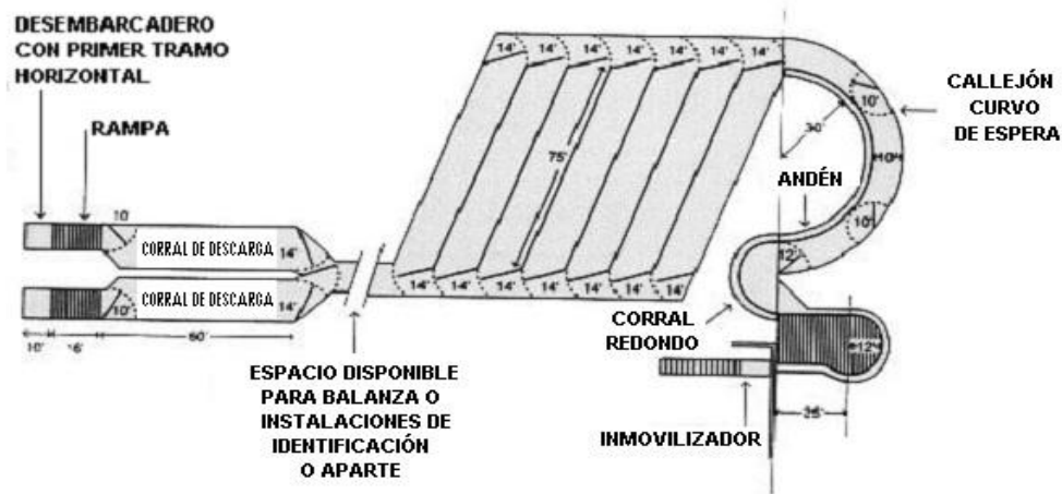
Esquema de distribución de manga de descarga y corrales de descanso
